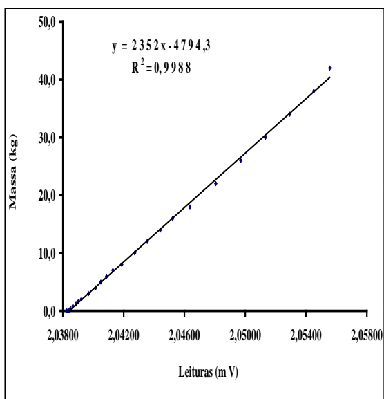
Figura 1. Resultados do ensaio de calibração de um lisímetro de pesagem obtidos com a adição das massas-padrão, em Limoeiro do Norte-CE, 2003.
