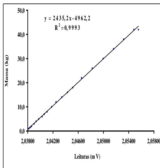
Figura 2. Resultados do ensaio de calibração de um lisímetro de pesagem obtidos com a subtração das massas-padrão, em Limoeiro do Norte-CE, 2003.
