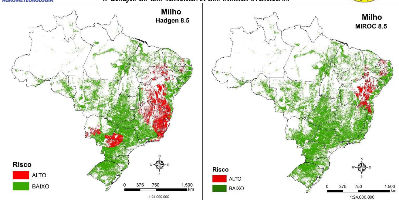
Figura 2. Áreas agrícolas agricultáveis do Brasil com a classificação de alto e baixo risco climático para a cultura do milho com base em dados do modelo regional ETA-HadGEN2-ES e ETA-Miroc5, RCP 8.5, para o período 2011-2040.
