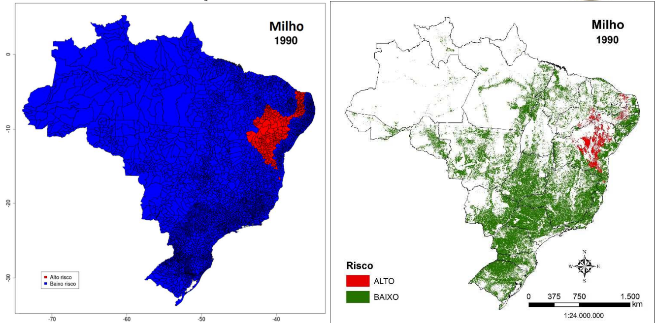
Figura 1. Classificação de alto e baixo risco climático para a cultura do milho no Brasil com base em dados do período 1976-2005 (1990 como ano central) (A) e áreas agrícolas agricultáveis de baixo e alto risco (B).
