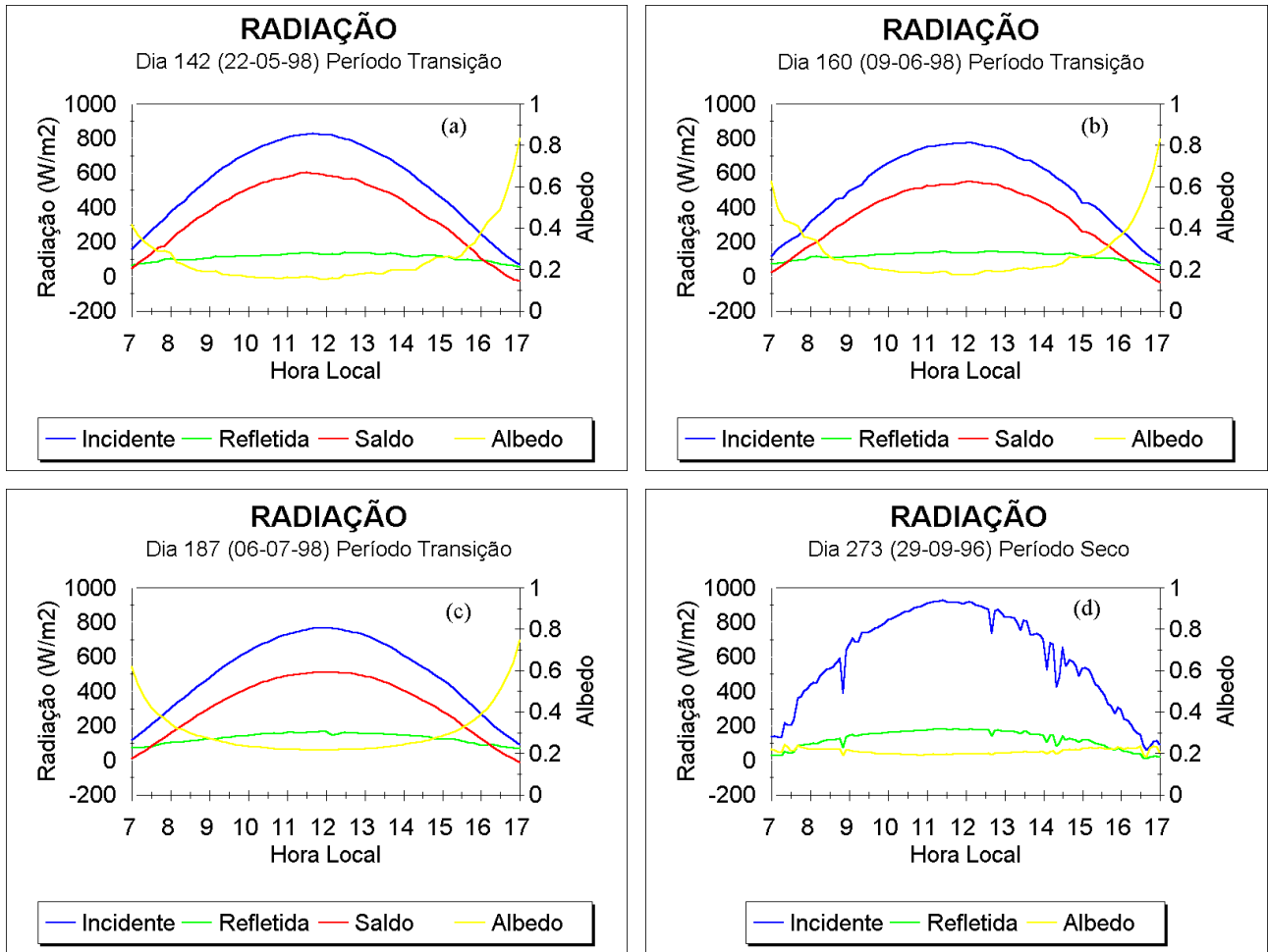
Figura 1 - Medidas de radiação e albedo nos períodos de transição/1998 (a-c) e seco/1996 (d).
