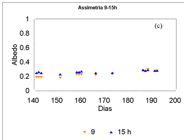
Figura 3 - Pareamento dos albedos matutinos e vespertinos no período de transição/1998:
