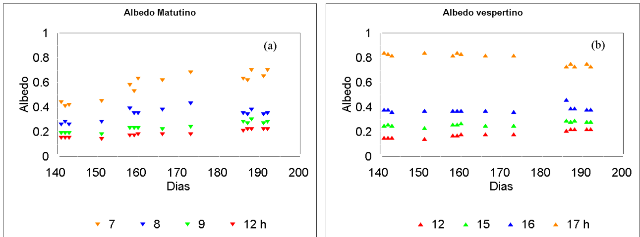
Figura 2 - Variação do albedo matutino (a) e vespertino (b) no período de transição/1998.
