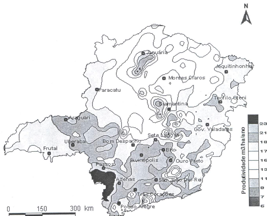
Figura 2. Potencial produtivo de eucalipto em Minas Gerais com o uso de médio nível tecnológico, obtido pelo modelo de crescimento 3-PG.
