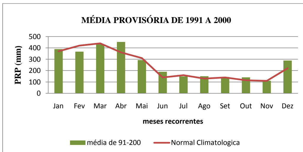
Gráfico 3-comparação entre a Normal climatológica e o sub-período de 91-00.
