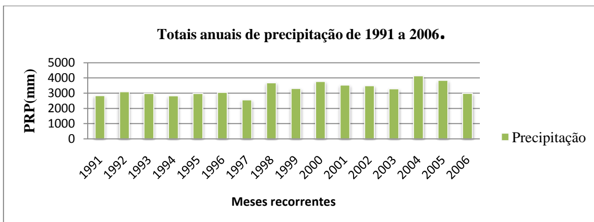
Gráfico 2- Total anual de precipitação (mm) desde 1991 a 2006.
