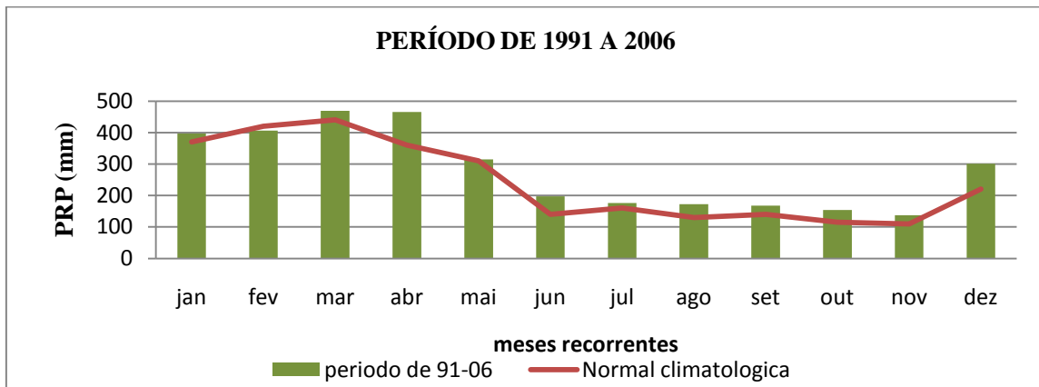
Gráfico 5-comparação entre valores da Normal 61-90 com o período de 1991 a 2006.
