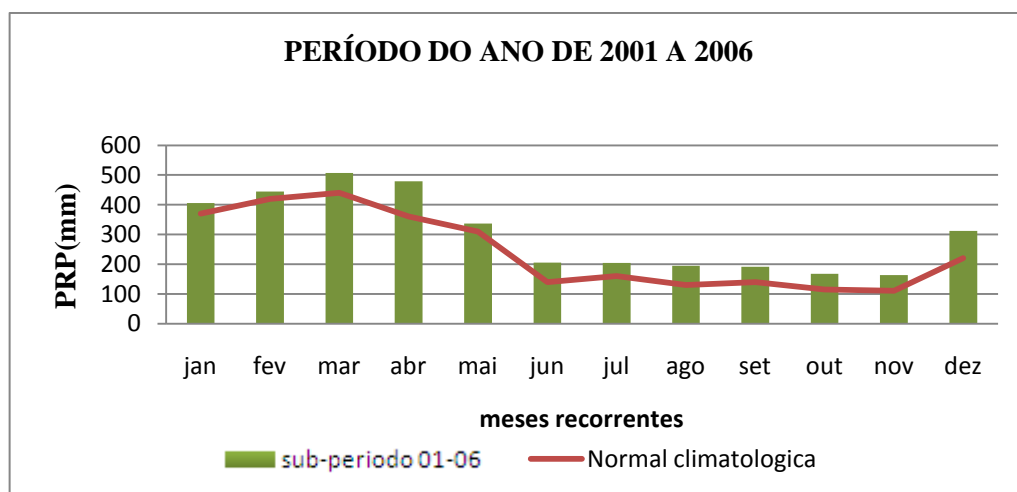
Gráfico 4-comparação entre valores da Normal 61-90 com o sub-período 01-06.
