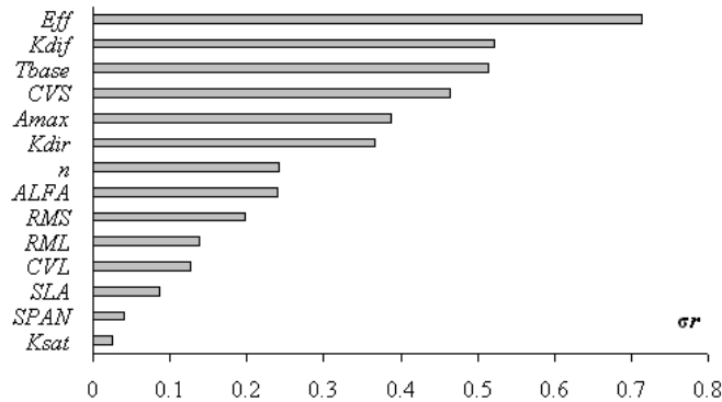
FIGURA 1 – Índice de sensibilidade relativa, em módulo e ordem decrescente, dos parâmetros analisados em função da variação de massa seca final da parte aérea ( \text{kg ha}^{-1} ) para o modelo SWAP/WOFOST parametrizado para cana-de-açúcar
