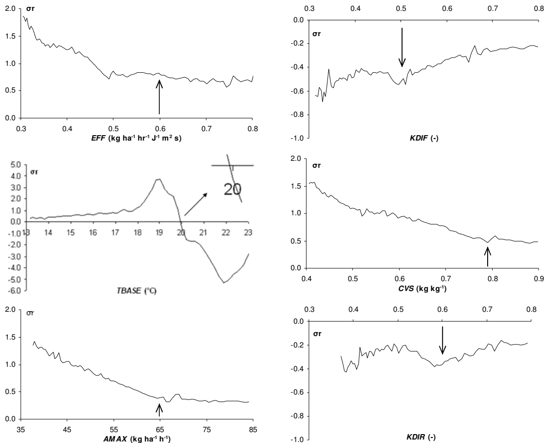
FIGURA 2 - Índice de sensibilidade relativa em função dos valores dos 6 parâmetros aos quais o modelo SWAP/WOFOST parametrizado para cana-de-açúcar é mais sensível.
