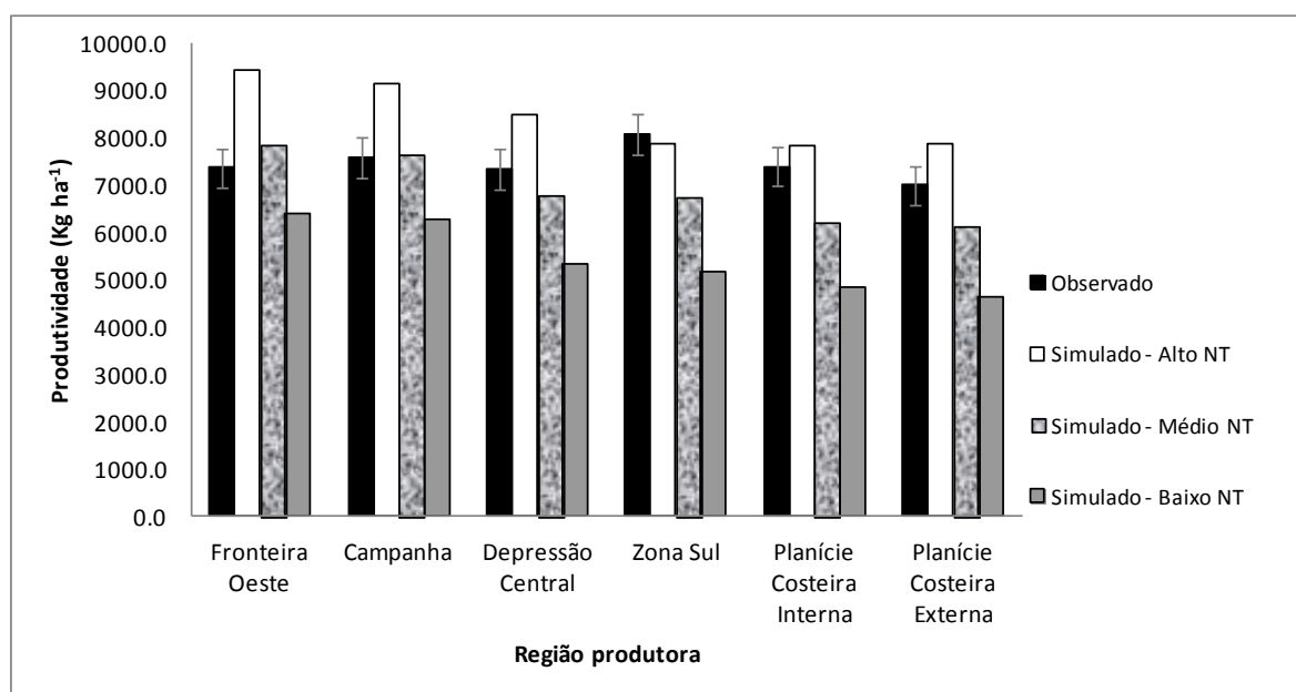
Figura 2. Produtividade média observada e simulada com o modelo SimulArroz em três Níveis de Tecnologia (NT) (alto, médio e baixo), para seis regiões produtoras de arroz do Rio Grande do Sul, na safra 2012/13.
