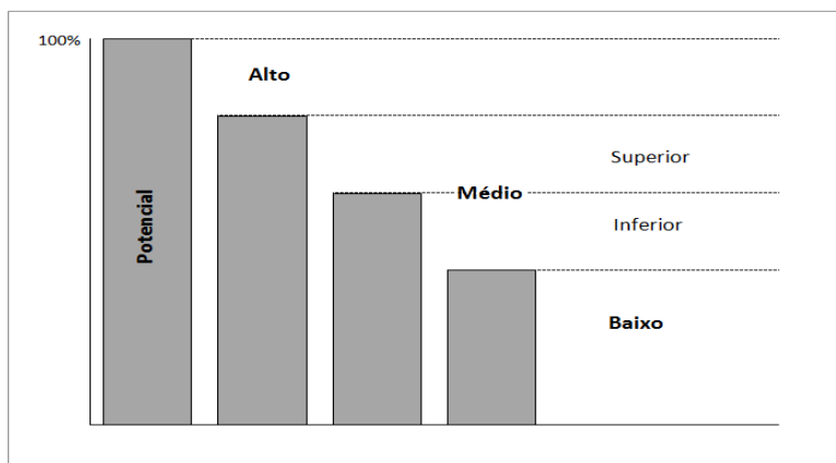
Figura 1. Níveis de tecnologia potencial, alto, médio e baixo, considerados no SimulArroz para a cultura do arroz irrigado no Rio Grande do Sul.
