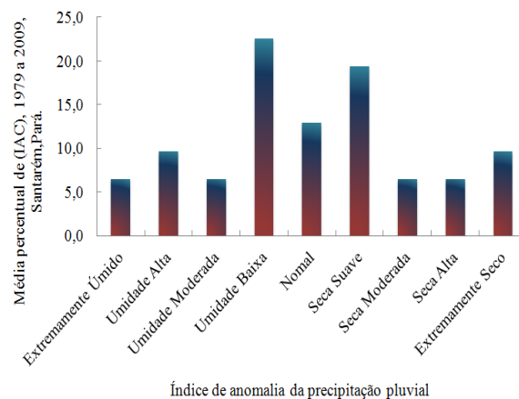
Figura 2. Média percentual de Padrões climáticos de umidade dos trinta e um anos observados em Santarém, Pará.
