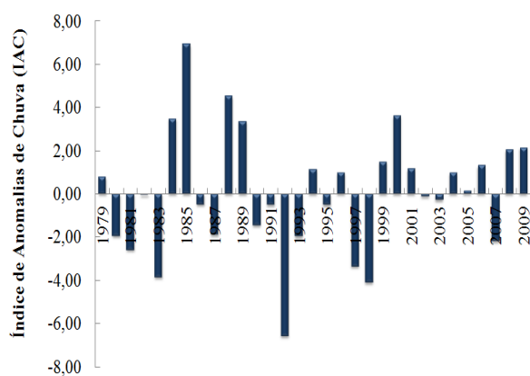
Figura 1. Índices de Anomalias de precipitação pluvial, correspondente ao período de 1979 a 2009 em Santarém, Pará.
