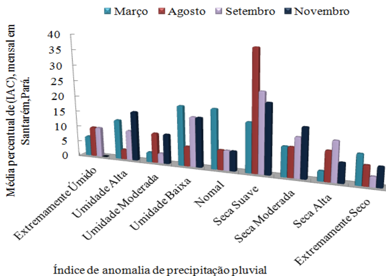
Figura 3. Média percentual mensal de padrões climáticos, da série histórica de 1979 a 2009, em Santarém, Pará.
