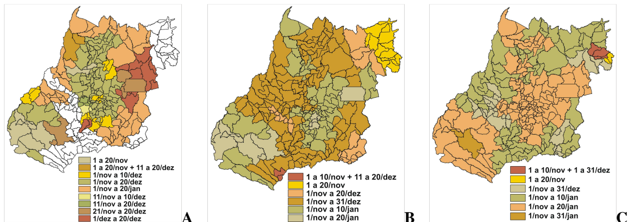
Figura 1. Caracterização de risco climático por deficiência hídrica (ISNA), para a cultura do milho consorciada com a brachiaria, considerando os solos Tipo 1 (A), Tipo 2 (B) e Tipo 3 (C), com capacidade de armazenamento de água de 20 mm, 40 mm e 60 mm, respectivamente.
