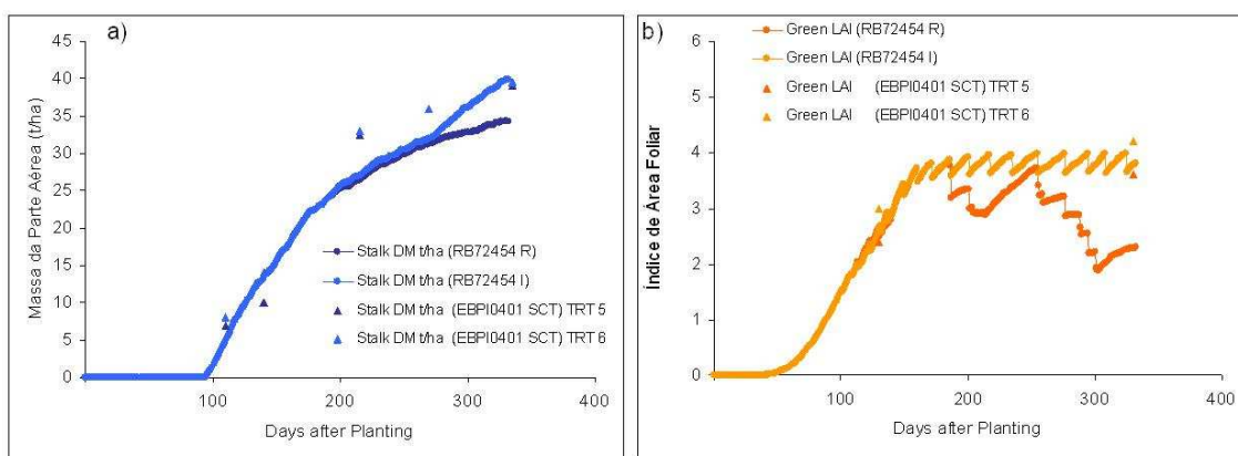
Figura 1. Variação diária da massa da parte aérea (a) e índice de área foliar (b) simulados pelo modelo Canegro e observados em condições de campo.
