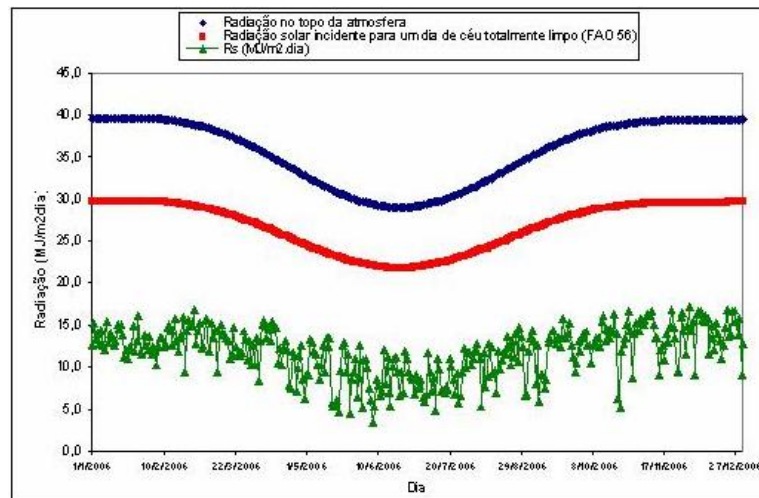
Figura 1 - - Radiação solar mensurada pela estação meteorológica automática (Metos, Pessl, Áustria), radiação solar no topo da atmosfera e a radiação solar incidente para um dia de céu totalmente limpo.
