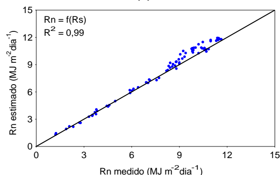
Figura 1. Validação dos modelos, apresentando a relação entre valores de radiação líquida (Rn) medida e estimada com base na temperatura média (T), temperatura máxima (TM), temperatura mínima (Tm), radiação global (Rs) e radiação extraterrestre (Ra).
